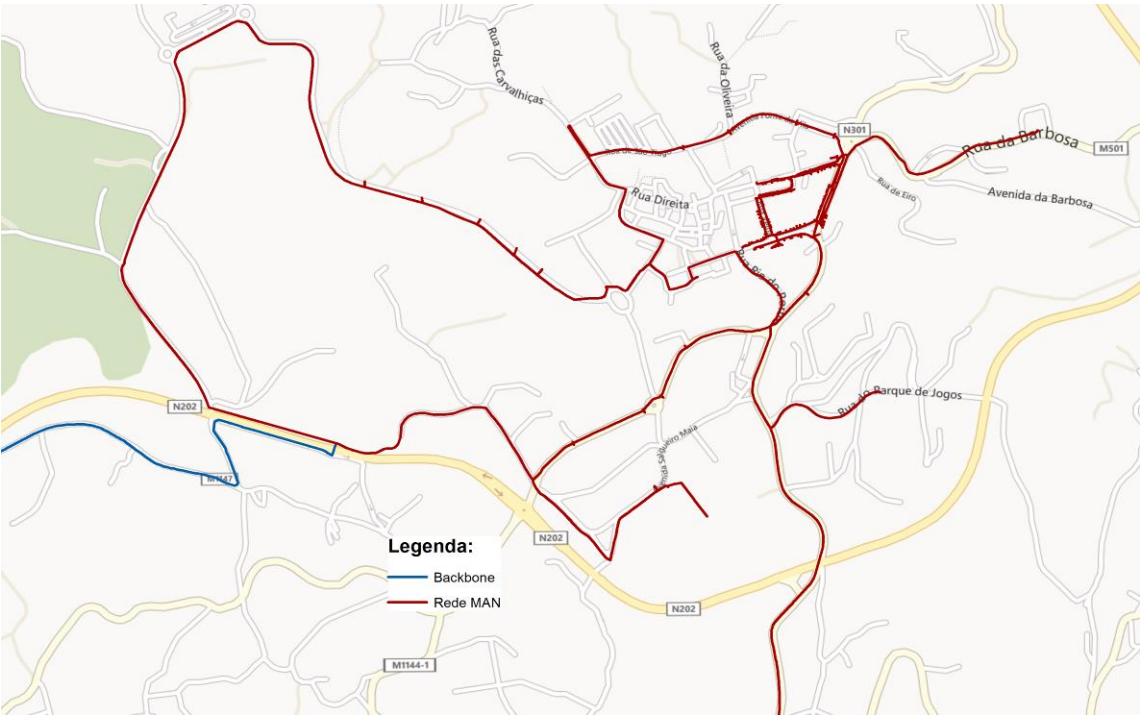
Fig.3 – Traçado da Rede MAN de Melgaço
