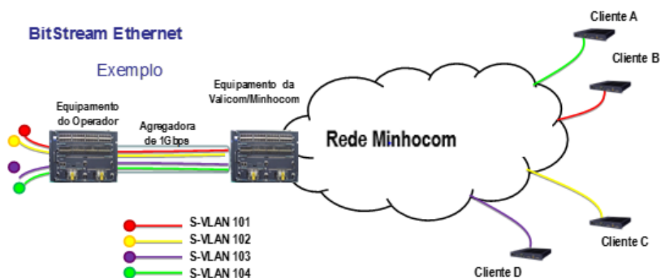
Figura 3: Arquitetura do Serviço BitStream Ethernet
