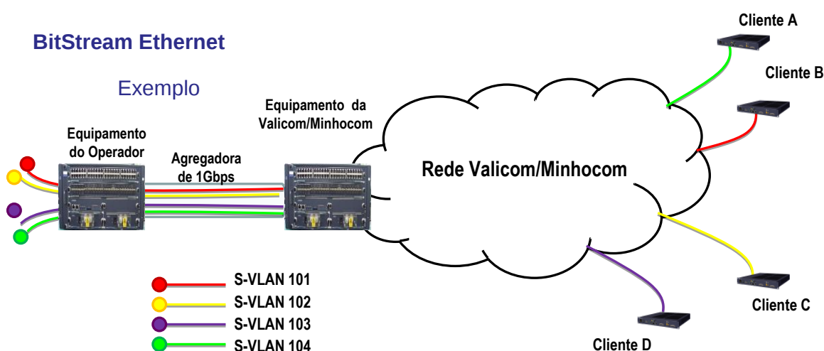
Figura 3: Arquitectura do Serviço BitStream Ethernet
