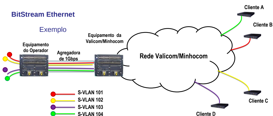
Figura 3: Arquitectura do Serviço BitStream Ethernet
