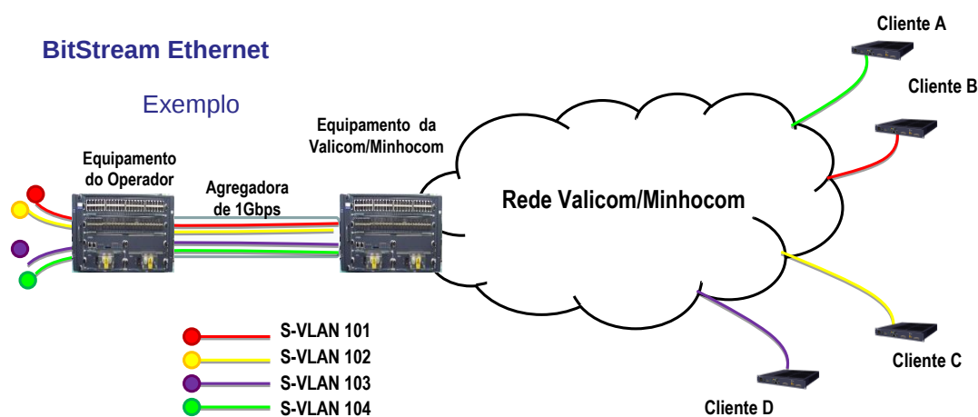
Figura 3: Arquitetura do Serviço BitStream Ethernet
